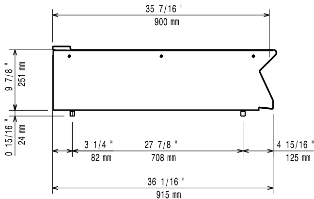
Boven aanzicht
